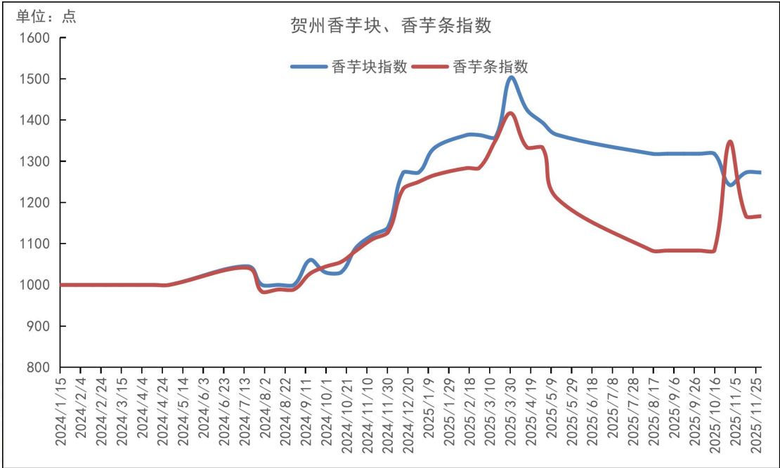
图 5 贺州香芋初级制成品价格指数走势
