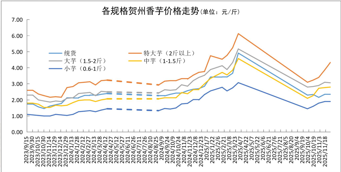
图 2 各规格贺州香芋价格走势
